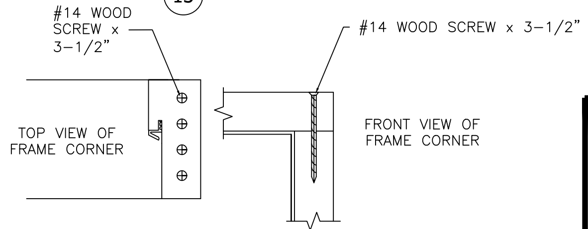
12 FRAME EDGE DETAIL
